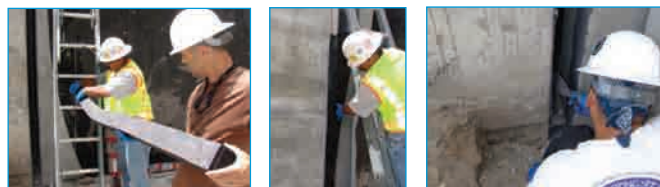
El sistema de 20H se instala desde el lado positivo de la pared de retención en una abertura de la junta preformada en concreto curado.
