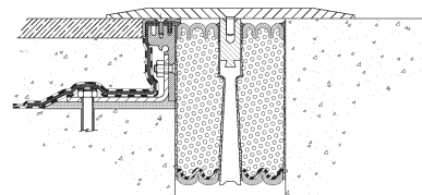
SJS-FP-FR también puede haber aplicaciones de cubiertas de doble losa a cubiertas de losa sólida. La presión posterior de la espuma SJS proporciona el anclaje y sellado requerido contra el lado sólido de la losa (a la derecha) de la junta de dilatación.
