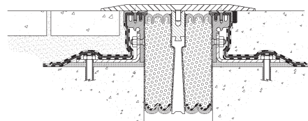
SJS-FP-FR ofrece una solución impermeable y resistente al fuego en situaciones de doble losa de cubierta a cubierta (arriba). Aquí se muestra una junta de dilatación junto con un sistema de junta de dilatación resistente al fuego instalado en un sustrato de hormigón (derecha) y una losa de hormigón con pavimento (izquierda)
