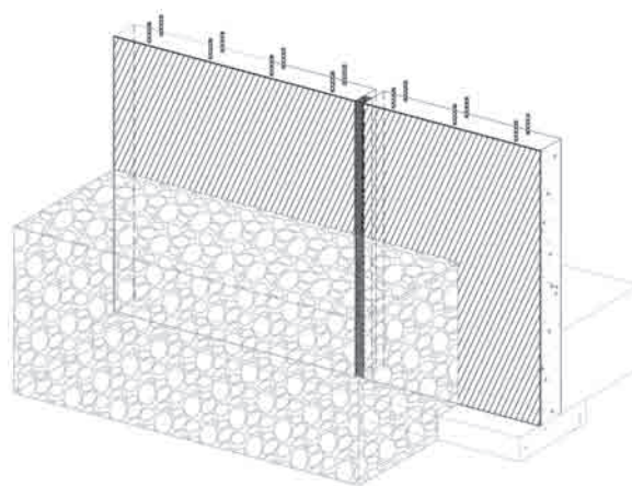
El Sistema de 20H en su lugar con un sistema de drenaje activo (suministrado por otros) para desviar el agua lejos de la fundación.
