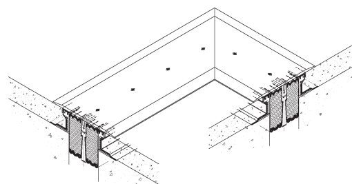
Transiciones herméticas transitables también se consiguen con el Sistema de SJS-FP-FR. Aquí se muestra una transición horizontal de 90 grados.
