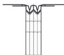
Sección transversal de RoofJoint sentada encima de la transición de la pared cerrada.
