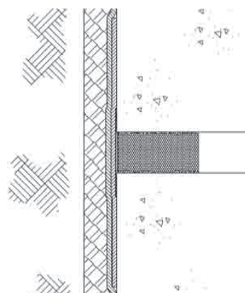
El Sistema 20H actúa como un apoyo resistente a las membranas impermeables por debajo del nivel.
